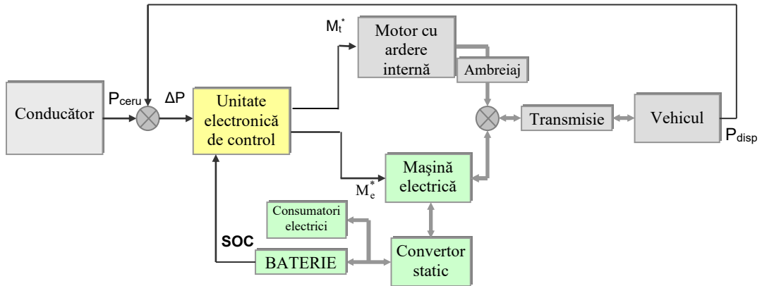
Figura 2. Modelul unui vehicul electric hibrid tip paralel.
