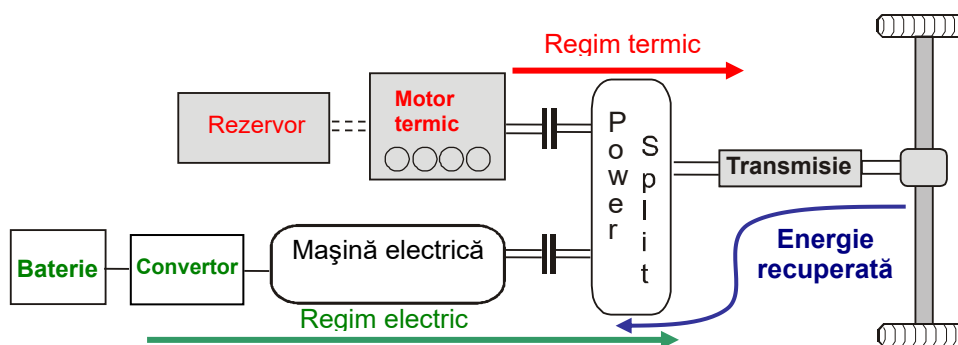
Figura 1. Structura unui vehicul electric hibrid de tip paralel.
